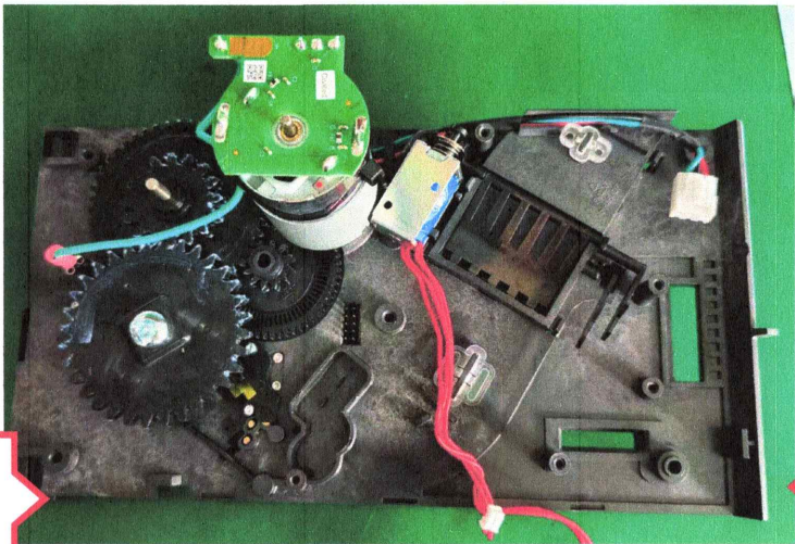
图一，识别 PA03163 组件，套上一个 NV200 PE 袋
